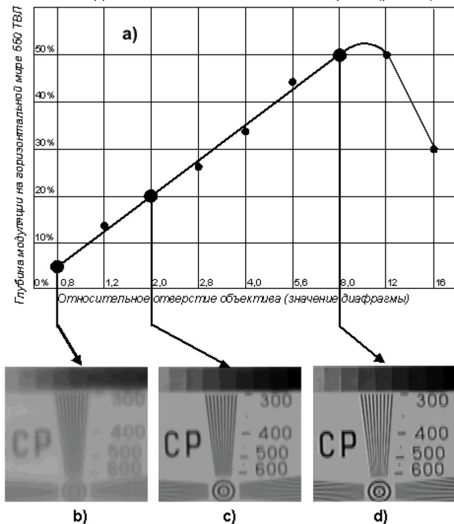
Рис. 17. Зависимость глубины модуляции сигнала (амплитуды частотно-контрастной характеристики) на горизонтальной мире 550 ТВЛ от относительного отверстия объектива (значения диафрагмы) в телевизионной камере высокого разрешения, при установленном объективе TO412FICS фирмы Computar.
