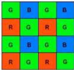
Три элемента, ухудшающие чувствительность цветных ПЗС камер: мозаичный фильтр, ИК отрезающий фильтр и процессор формирования цветного сигнала (слева направо)
